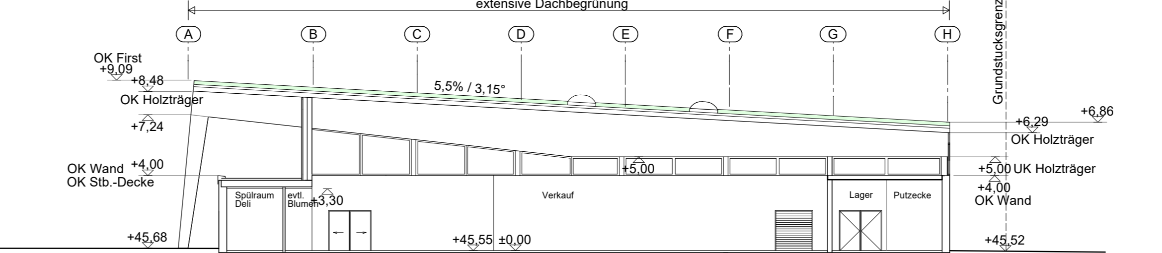
Querschnitt
