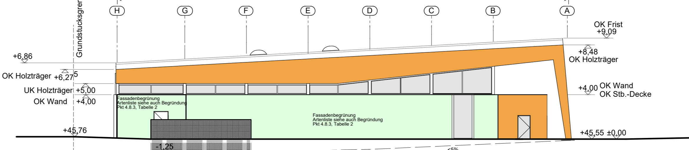
Ansicht Südwest
