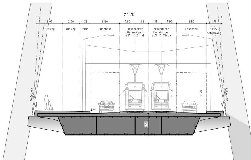
REGELQUERSCHNITT ALTE ELBE - VARIANTE 6
