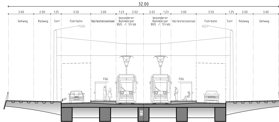
REGELQUERSCHNITT ZOLLELBE - VARIANTE 6
