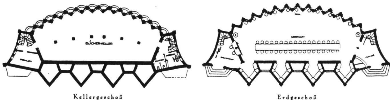
Projekt Gefallenendenkmal von Bruno Taut, Grundrisse
